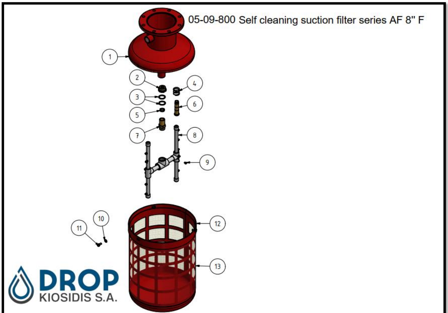
*05-09-800 Filtr série AF 8" samočistící sací filtr
