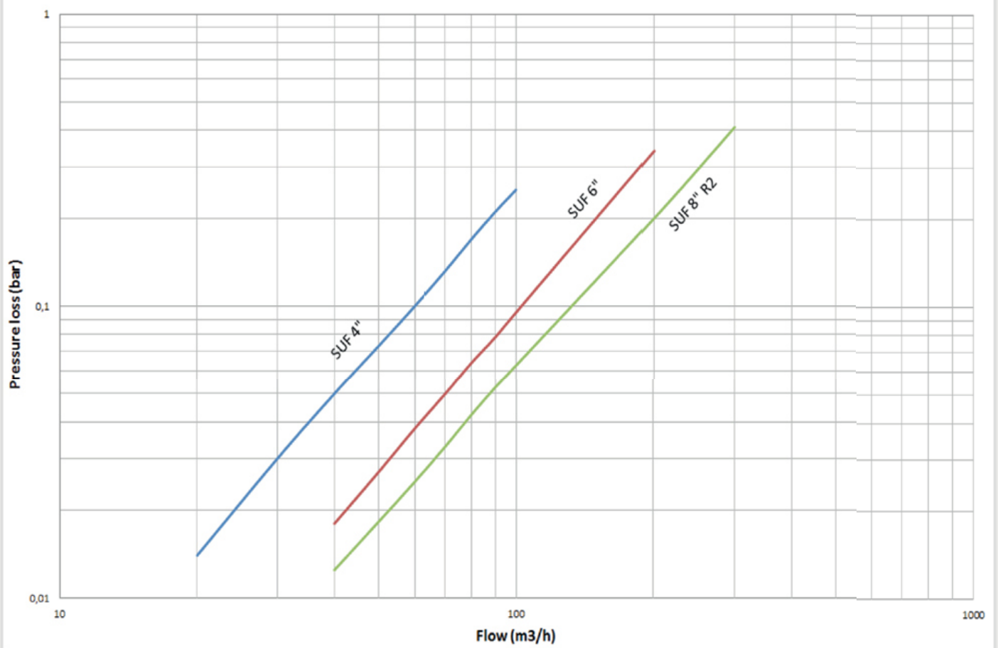
HEADLOSS SUF
