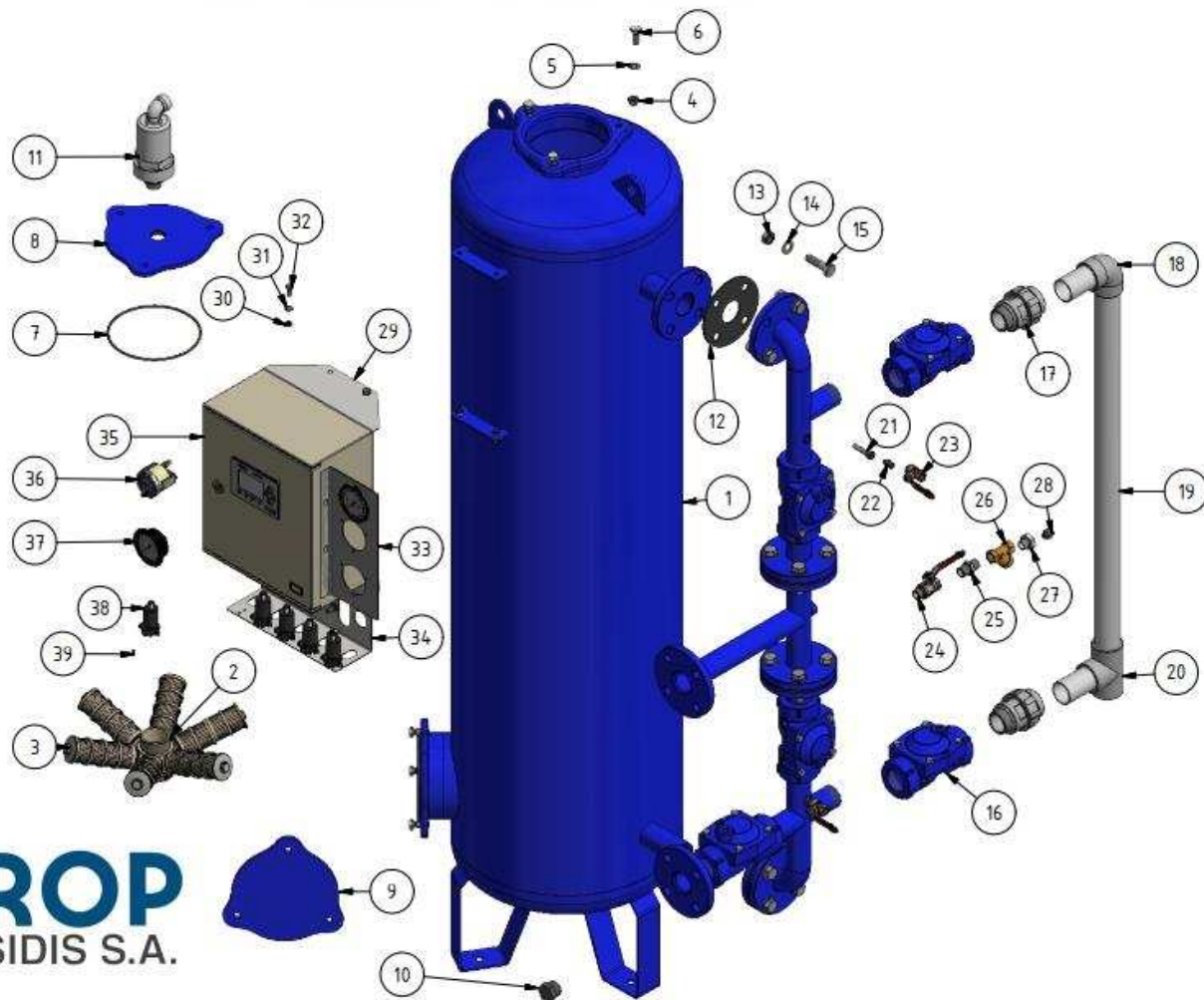
02-17-152 Filtr s různými čisticími prostředky série WTX 1 1/2"-18" Auto
